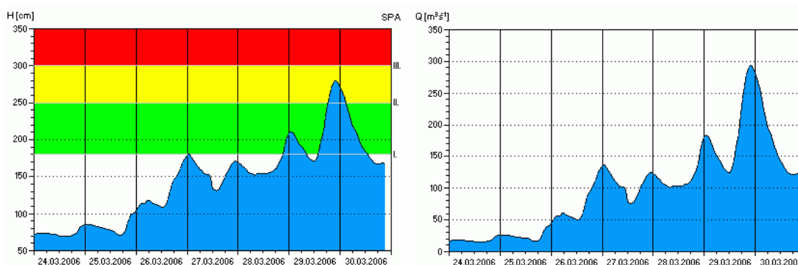
Graf výšky hladiny (vlevo) a průtoku (vpravo) na Olši.
