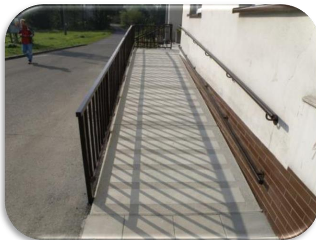
Oprava vstupu do budovy Domu s pečovatelskou službou čp. 670
